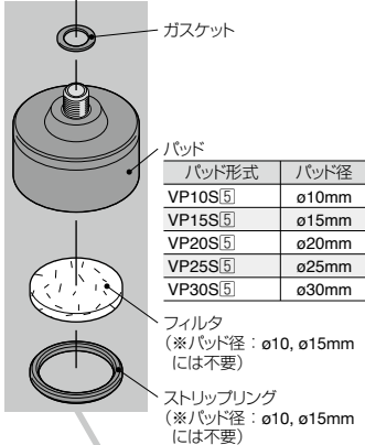
パッド直付タイプフィルタ
