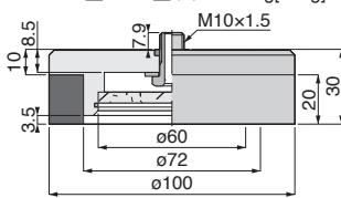
VP100S③-M10⑨ 質量：272g[300g]
