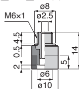
VP10S③-M6⑨ 質量：1.9g[1.9g]
