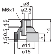
VP15S③-M6⑨ 質量：2.1g[2.3g]
