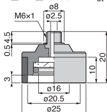
VP50S③-M6⑨ 質量：76g[83g]
