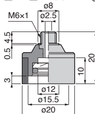
VP35S③-M6⑨ 質量：35g[40g]
