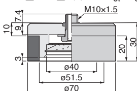
VP70S③-M10⑨ 質量：142g[156g]
