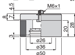
VP50S③-M6⑨ 質量：76g[83g]
